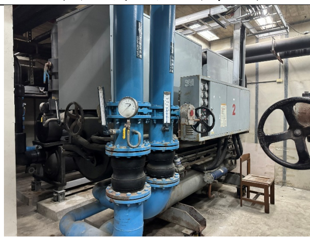
113 年東海大學圖書館；總工程款 1848.5 萬，補助款 500 萬，節能率 49.2%。 工程內容汰換 300RT 冰水主機*2 台及附屬設備。
